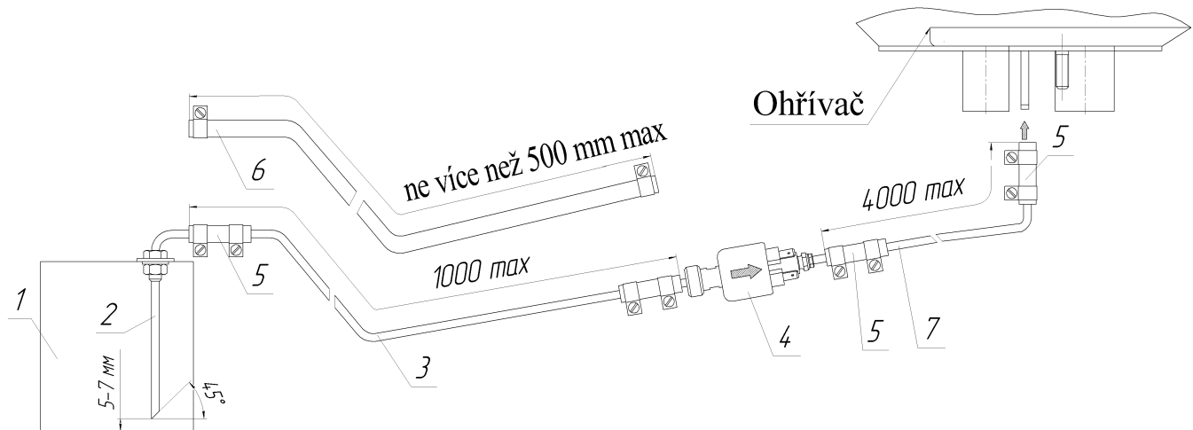
Obr. č. 8.5 - Instalace zařízení pro přívod paliva.
